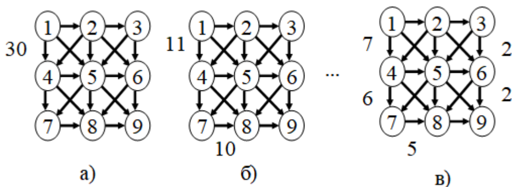
Рисунок 5 – Второй пример реализации полносвязных кластерных многопроцессорных систем с соответствующими вариантами размещения
