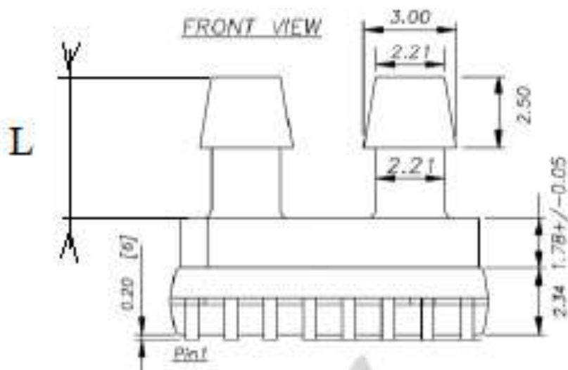
Рисунок 3 – Внешний вид датчика динамического давления
