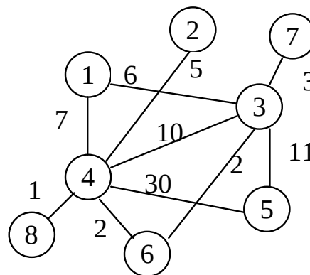
Рисунок 1 – Граф задачи
