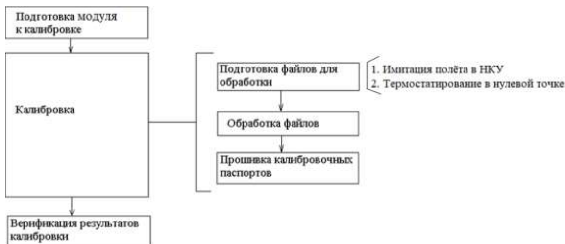
Рисунок 1 – Этапы калибровки датчиков СВС
