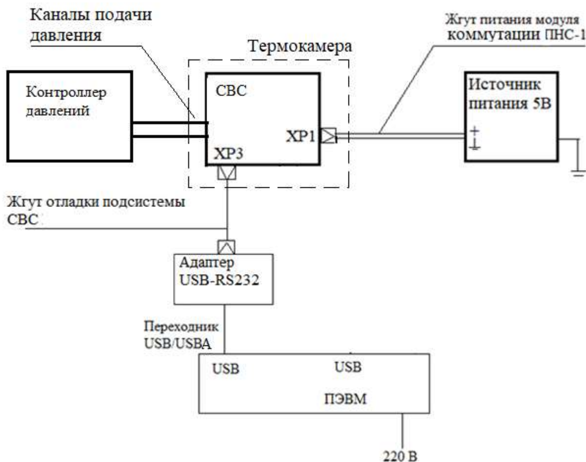
Рисунок 4 – Схема подключения модуля коммутации при проведении калибровки
