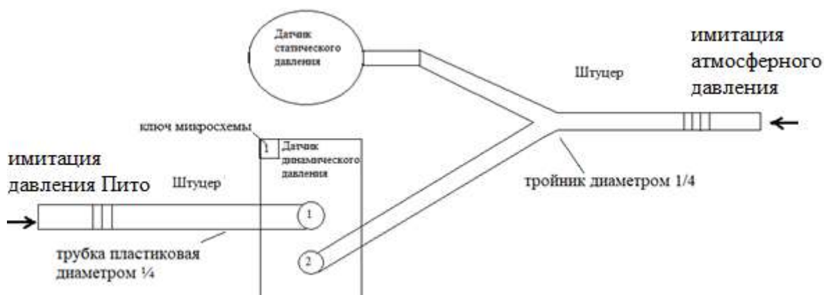
Рисунок 2 – Схема соединения патрубков датчиков с тестером воздушных сигналов ADTS42F
