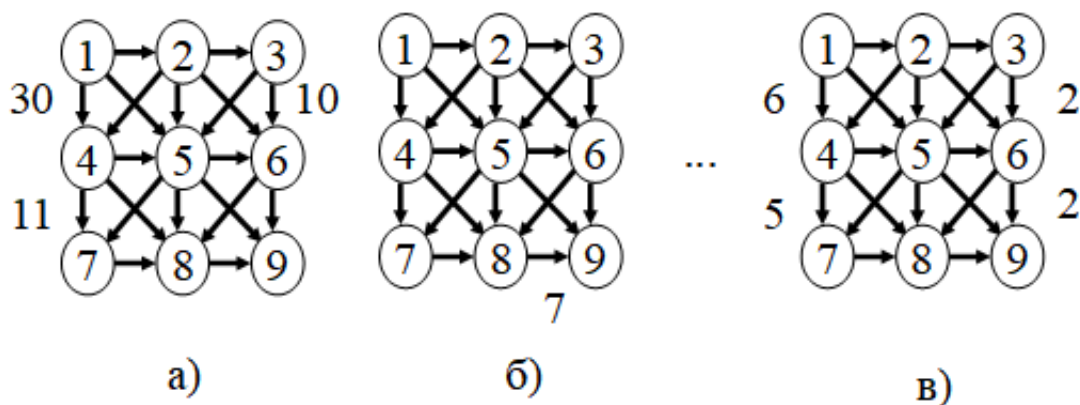
Рисунок 4 – Первый пример реализации полностью связанных кластерных многопроцессорных систем с соответствующими вариантами размещения
