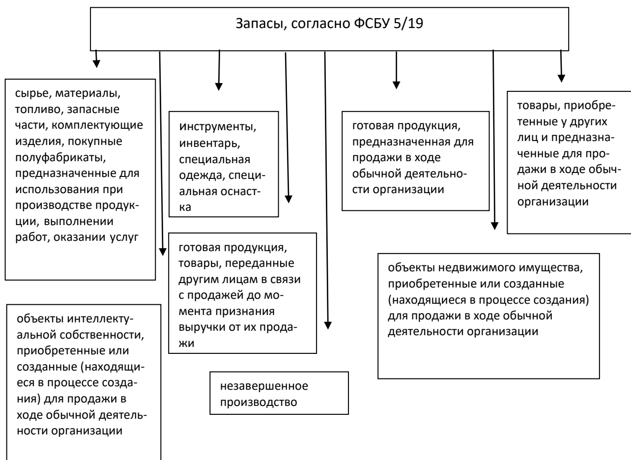
Рисунок 2 – Классификация запасов
